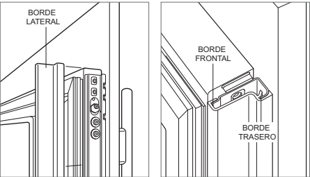
Borde de la puerta Bordes del soporte
