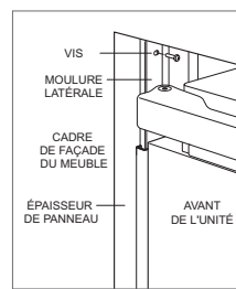
Ancrage
