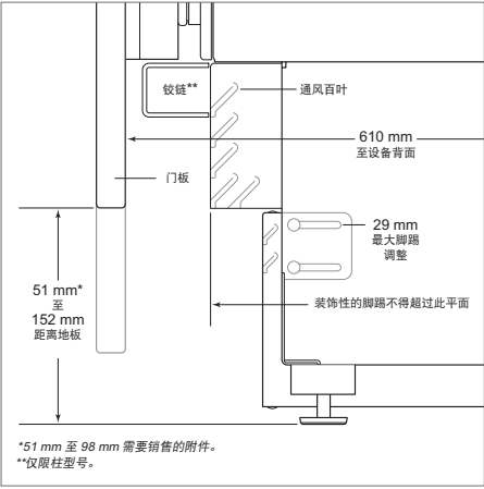
脚踏（侧视图）
