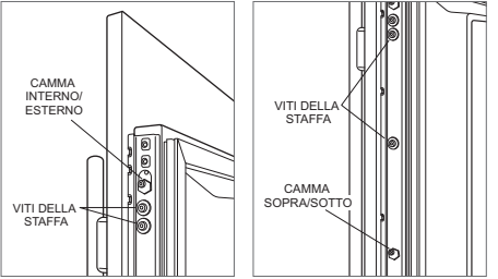
regolazione interno-esterno regolazione su e giù
