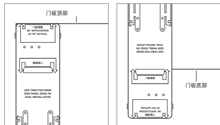
门板模板一顶部
