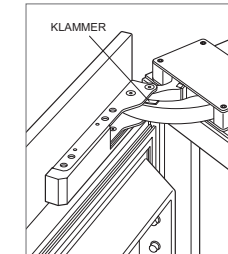
Türanschlag von 90°
