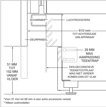
Teenstootplaat (zijaanzicht)
