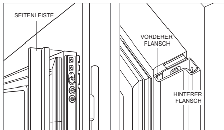
Seitliche Türeinfassung
