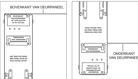
Sjabloon deurpaneel: bovenkant Sjabloon deurpaneel: onderkant (hoog model)
