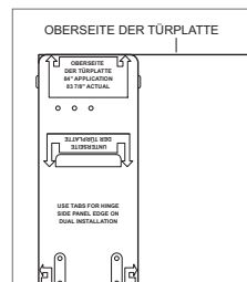
Türplattenvorlage – oben
