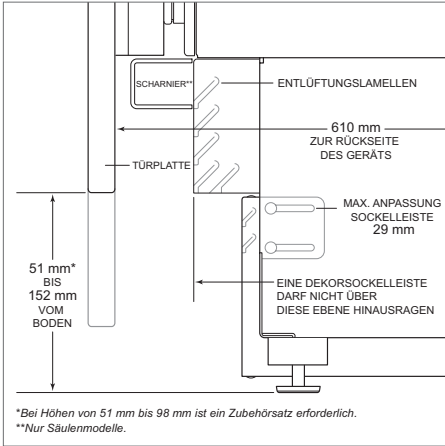
Sockelleiste (Seitenansicht)
