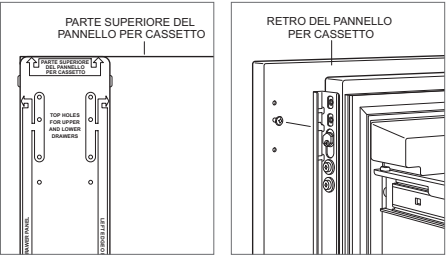
Mascherina del pannello del cassetto—superiore Montaggio del pannello del cassetto
