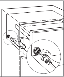
Cable de control (modelo de cajón)
