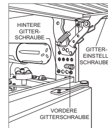
Gitterhöheeneinstellung
