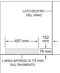
Posizione dell'alimentazione dell'acqua
