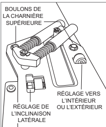
Boulons de réglage de la porte
