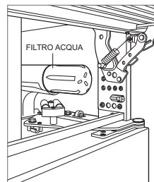
Rimozione del filtro dell'acqua
