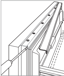
Borde superior del cajón
