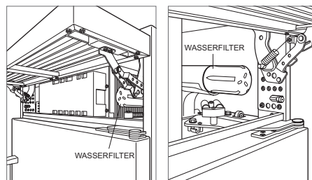
Einbauort des Wasserfilters
