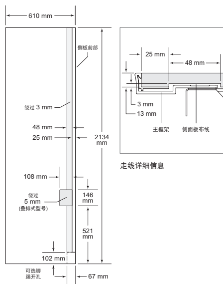
側面板尺寸
