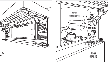
格栅拆卸
