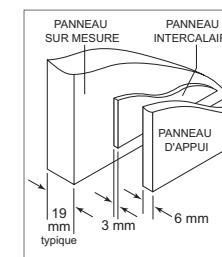
Vue arrière de l'assemblage des panneaux
