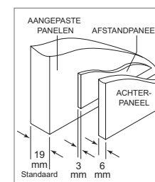
Paneelmontage (achteraanzicht)
