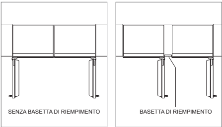
Cardini opposti Cardini sullo stesso lato
