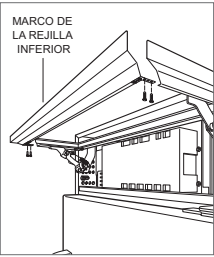
Conjunto del marco de la rejilla
