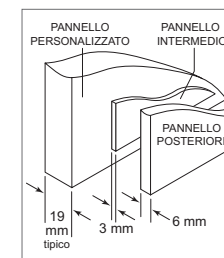
Vista posteriore gruppo pannelli
