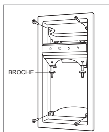
Retrait de l'encadrement du distributeur
