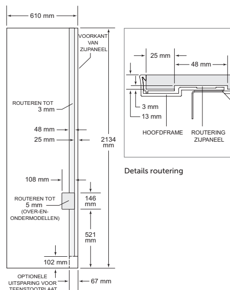
Afmetingen zijpaneel
