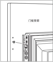
门板安装
