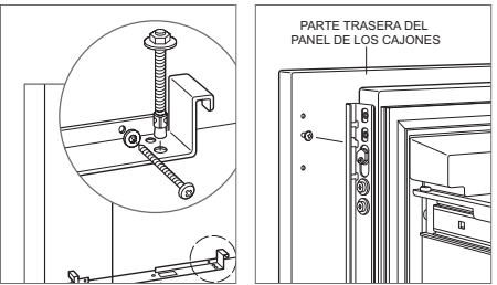
Plantilla del panel del cajón: parte superior Montaje del panel del cajón
