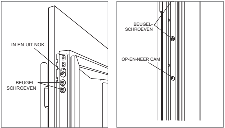
Aanpassing in-en-uit Aanpassing op-en-neer
