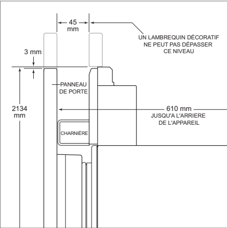
Lambrequin supérieur (vue latérale)
