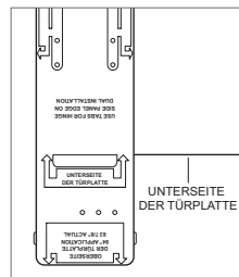
Türplattenvorlage – unten (nur hohe Modelle)
