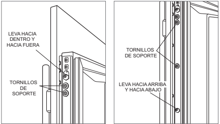
Ajuste hacia dentro y hacia fuera Ajuste hacia arriba y hacia abajo
