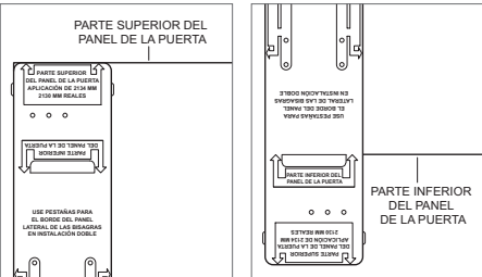
Plantilla del panel de la puerta: parte superior Plantilla del panel de la puerta: parte inferior (solo modelos altos)
