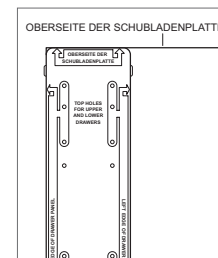
Schubladenplattenvorlage – oben
