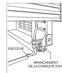
Canalisation d'eau
