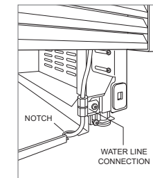
Watertoevoerslang
