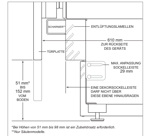
Sockelleiste (Seitenansicht)
