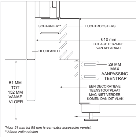
Teenstootplaat (zij aanzicht)
