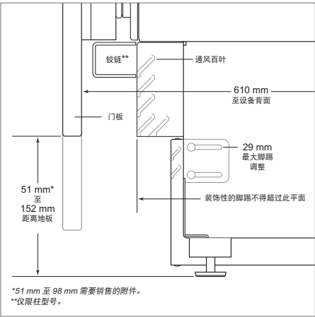
脚踢（侧视图）
