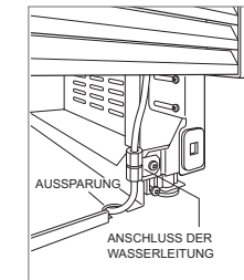
Wasserleitung
