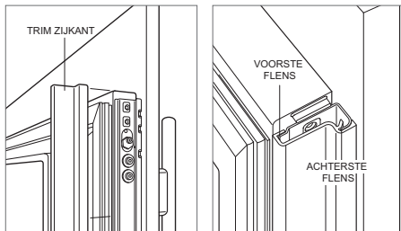
Deurtrim zijkant
