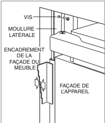
Ancrage
