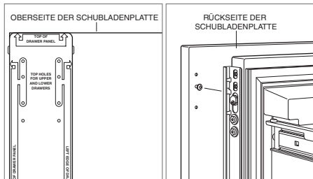
Schubladenplattenvorlage – oben
