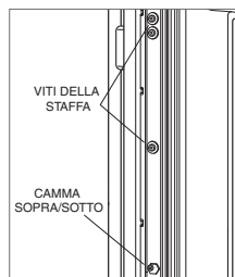
Regolazione verticale delle porte
