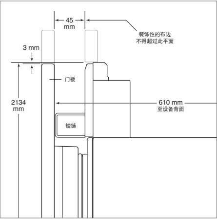
上部窗帘框（柱和高型号）—侧视图。
