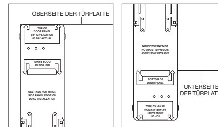
Türplattenvorlage – oben
