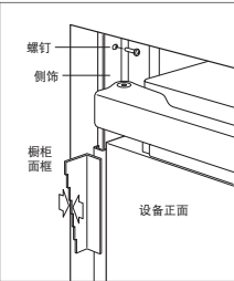
锚定。
