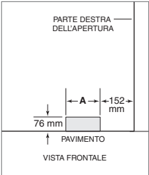
Posizione della conduttura dell'acqua
