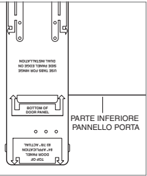
Dima pannello porta, parte inferiore (solo modelli a colonna)
