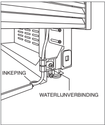
Waterleiding.
