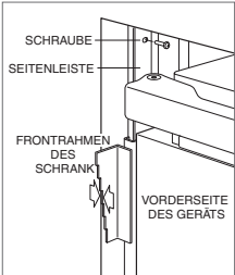
Verankerung
