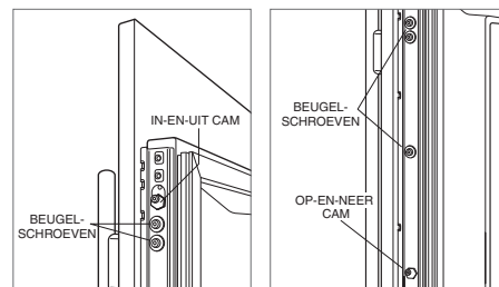
Aanpassing in-en-uit
