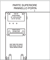
Dima pannello porta, parte superiore
