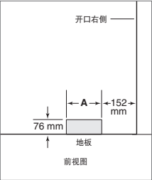
供水位置。
