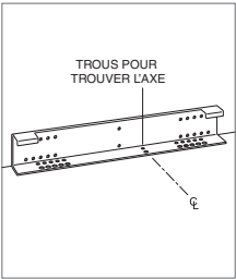
Support antibascullement
