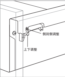
抽屉调节
