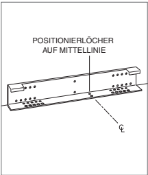
Kippschutzhalterung
