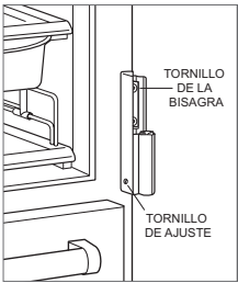
Ajuste de la bisagra del armario
