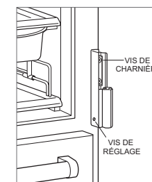
Ajustement de la charnière de meuble
