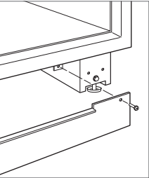
踢脚板安装
