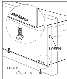
Schubladenneigungseinstellung
