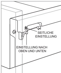
Schubladeneinstellung
