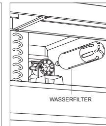
Wasserfilter entfernen
