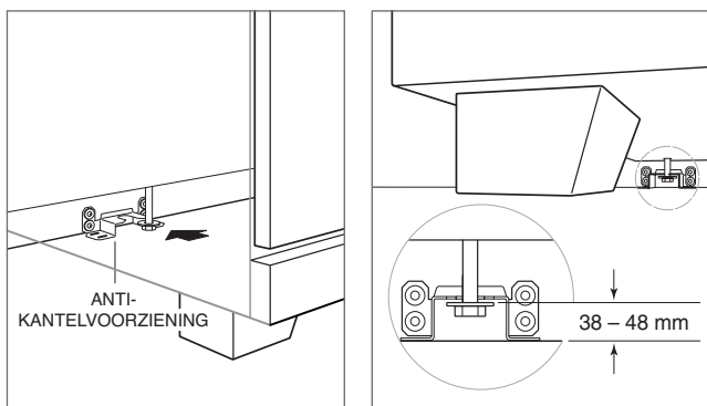
Locatie anti-kantelvoorziening Anti-kantelvoorziening in werking
