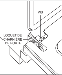
Démontage de la porte du four
