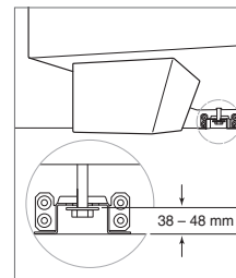
Bullone antiribaltamento agganciato
