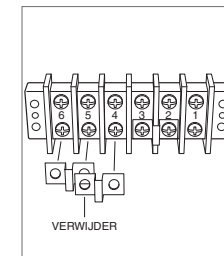
3-fasig
