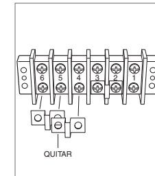
Cableado trifásico
