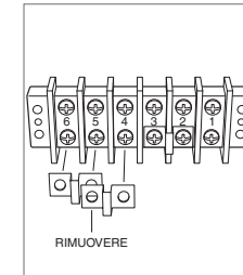
Trifase
