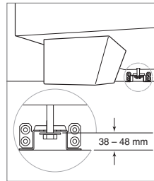
Kippschutzbolzen eingerastet
