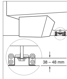
Anti-kantelbout gekoppeld
