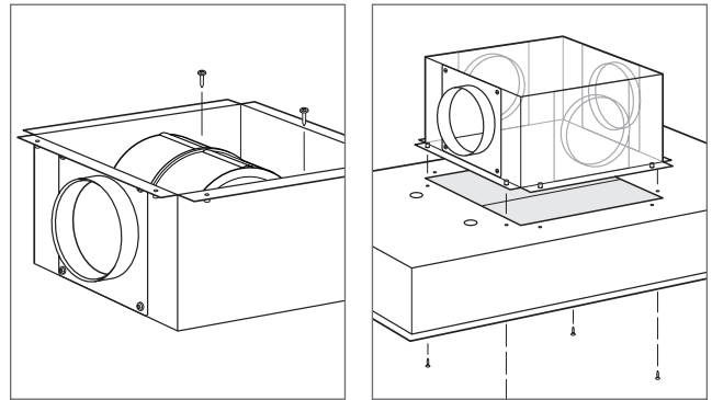
Instalación del extractor interno Dirección de la descarga
